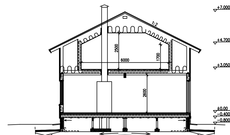
LEVENNETTY + KOROTETTU 60 cm 6 m LATTIA KATTOKALTEVUUS 1:2
